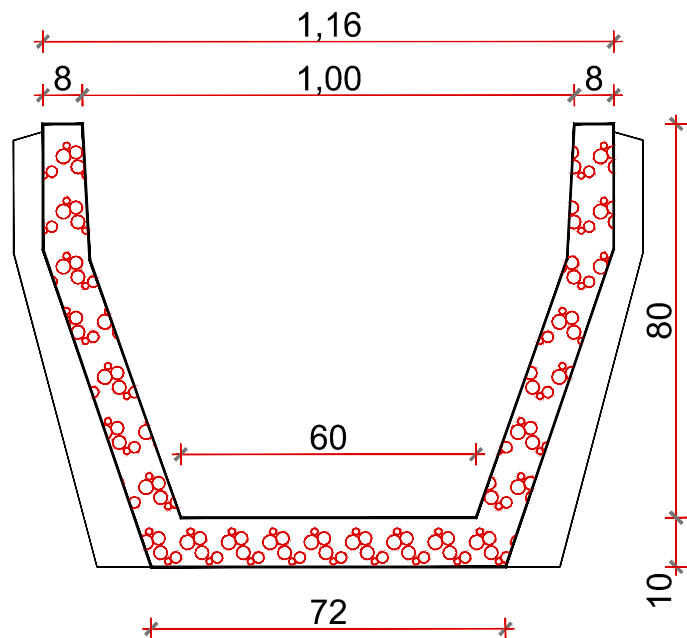
KERESZTMETSZET
